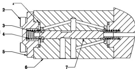
图二 电磁阀结构示意图
