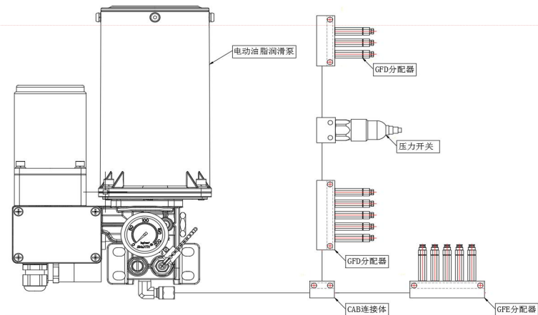
容积式系统示意图
