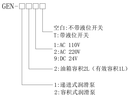
油箱式润滑泵
