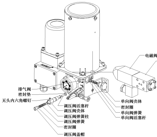
图一 润滑泵结构示意图
