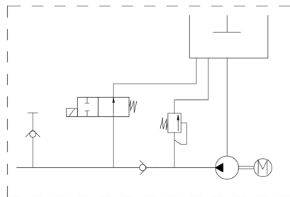
容积式式原理图
